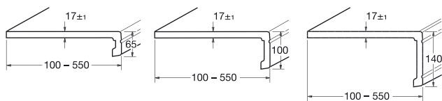
Стандартная высота капиносов системных подоконников
