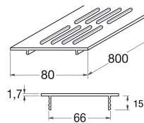
Вентиляционная решетка
