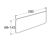
Торцевая заглушка для системных подоконников с наращенным капиносом
