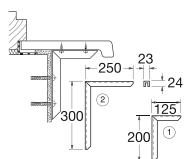
Кронштейны
