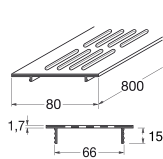
Вентиляционная решетка
