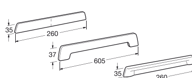
Торцевая заглушка exclusiv
