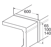
Соединительный профиль
