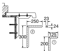
Кронштейны
