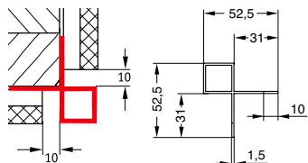
Алюмінієвий зовнішній кутвий профіль
