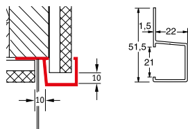
З'єднувальний профіль F
