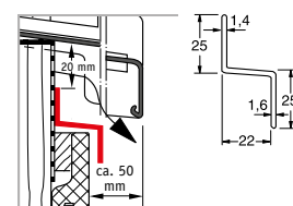
Z-профіль 2
