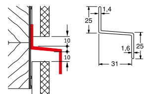
Z-профіль 1
