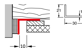
Внутрішній куточок 30/20
