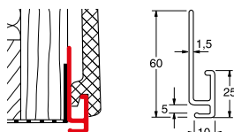
Початковий профіль N + F
