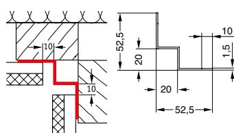
Алюмінієвий внутрішній кутвий профіль
