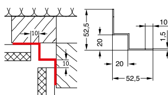
Алюминиевый внутренний угловой профиль
