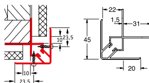
Внешний уголок C
