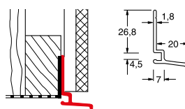
Начальный профиль для вертикального монтажа
